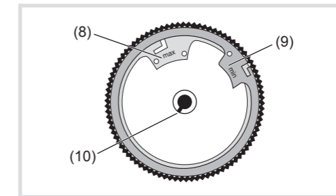
Afb. 5: Regelknop achteraanzicht
