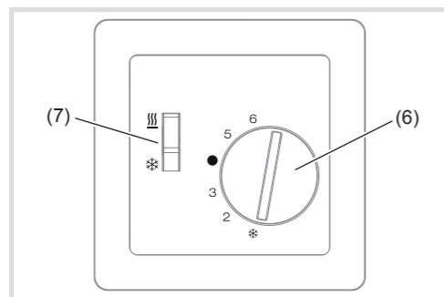
Afb. 2: Bedieningselementen
